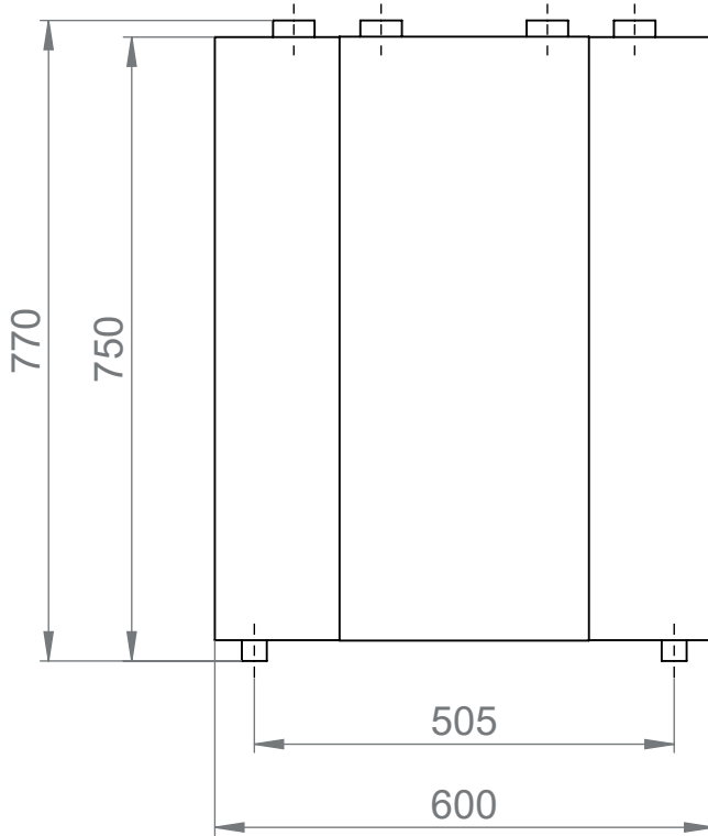
Frontansicht
